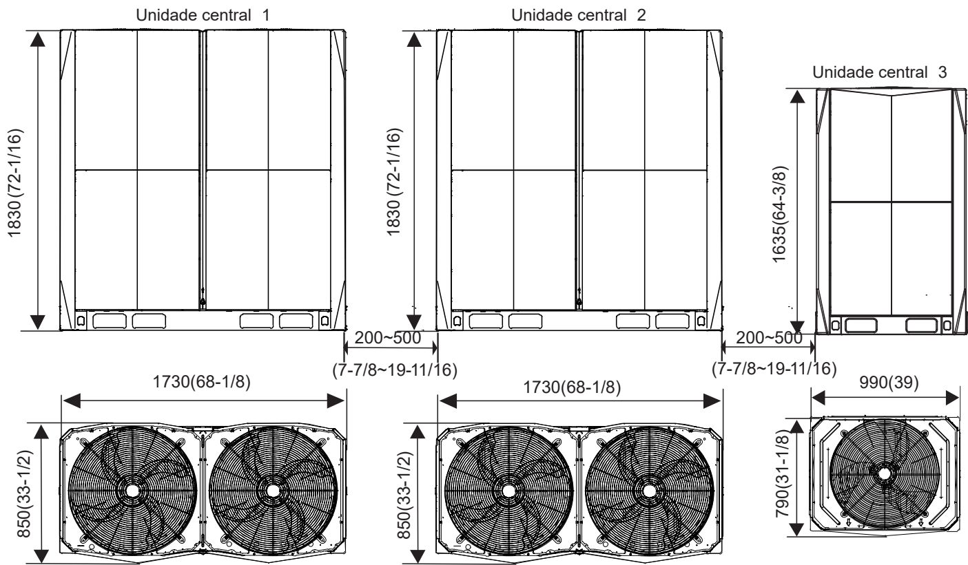
Figura 2-2.11: Dimensões da unidade 68HP (unidade: mm (polegada))
