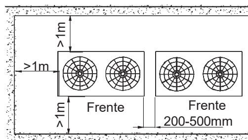
Figura 3-2.3: Instalação em várias filas (unidade: mm)
