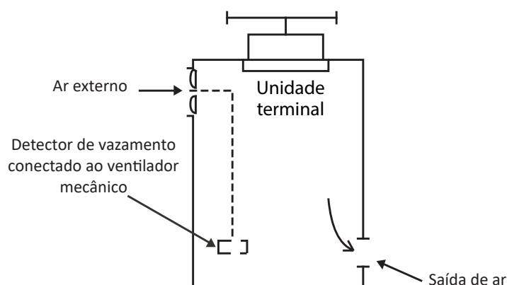
Figura 3-4.8: Ventilador mecânico controlado pelo detector de vazamento de refrigerante
