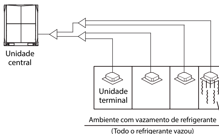
Figura 3-4.7: Cenário potencial de vazamento de refrigerante
