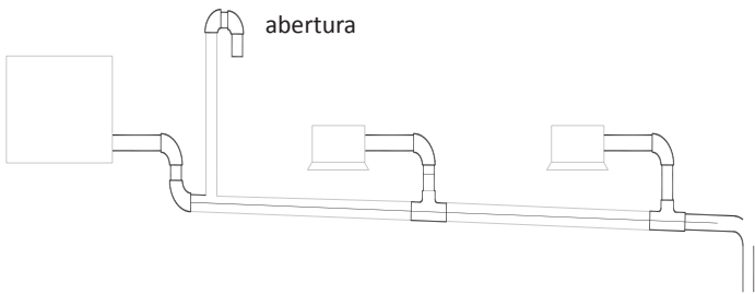
Figura 3-6.5: Saídas de ar dos tubos de drenagem
