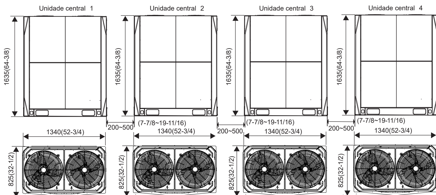
Figura 2-2.23: Dimensões da unidade 86/88*HP (unidade: mm (polegada))
