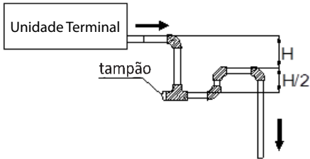
Figura 3-6.6: Coletores de água da tubulação de drenagem
