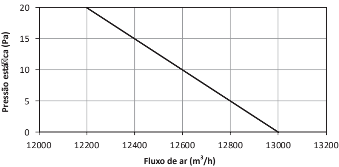
Figura 3-3.8: Desempenho do ventilador 14-16HP
