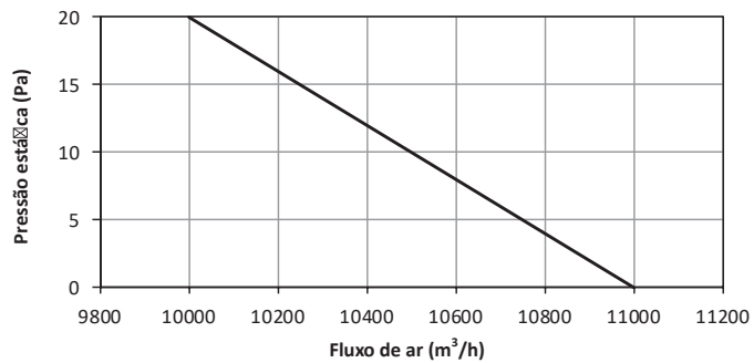
Figura 3-3.7: Desempenho do ventilador 8-12HP
