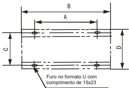
Figura 3-2.6: Posicionamento do parafuso de expansão
