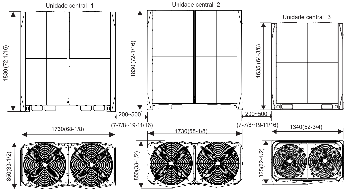
Figura 2-2.12: Dimensões da unidade 70/72/74/76/78HP (unidade: mm (polegada))
