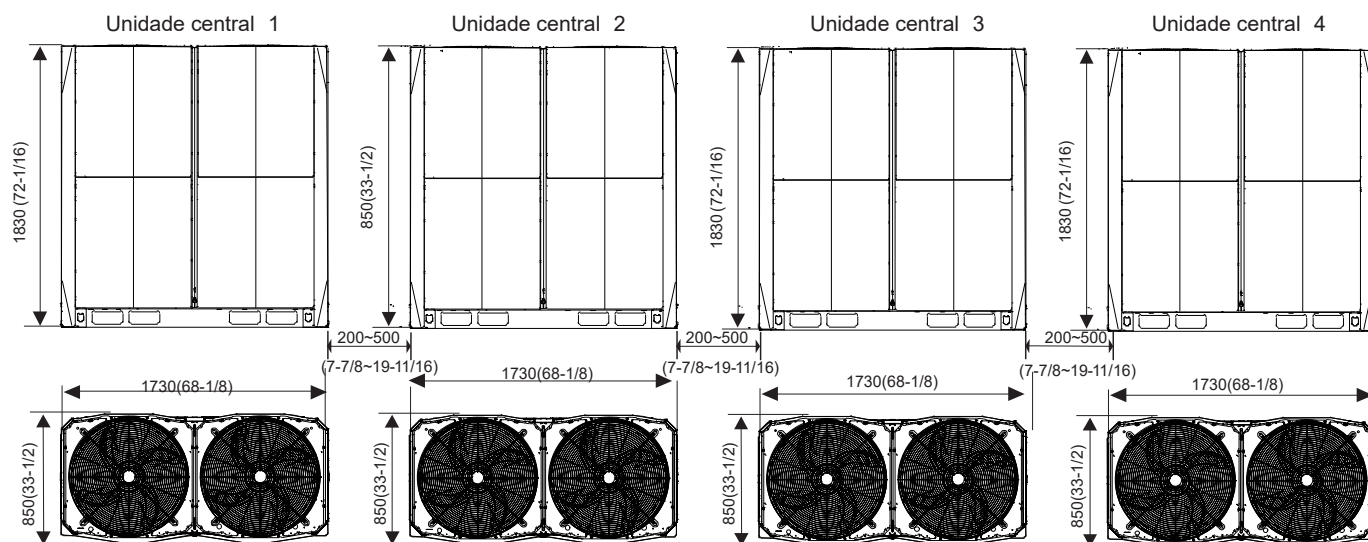
Figura 2-2.15: Dimensões da unidade 96*HP (unidade: mm (polegada))
