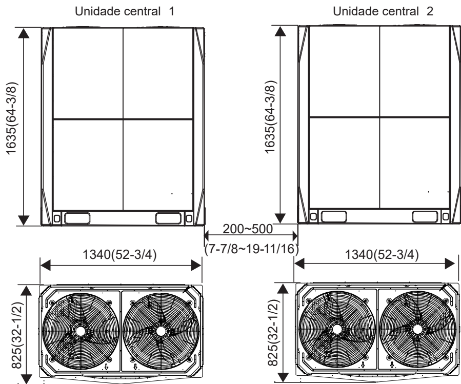
Figura 2-2.16: Dimensões da unidade 30/32/36HP (unidade: mm (polegada))
