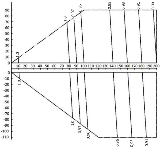
Figura 2-8.2: Taxa de alteração na capacidade de aquecimento
