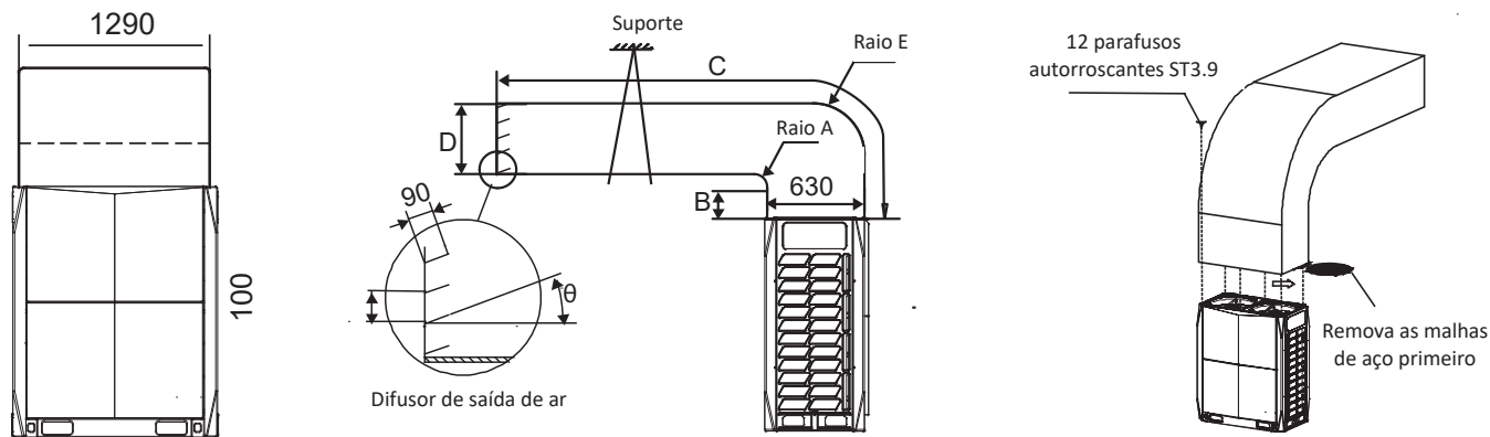
Figura 3-3.4: Duto transversal para unidades de 14HP-22HP (unidade: mm)
