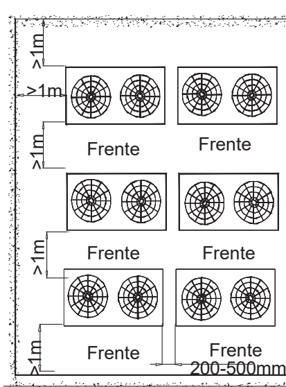
Figura 3-2.3: Instalação em várias filas (unidade: mm)
