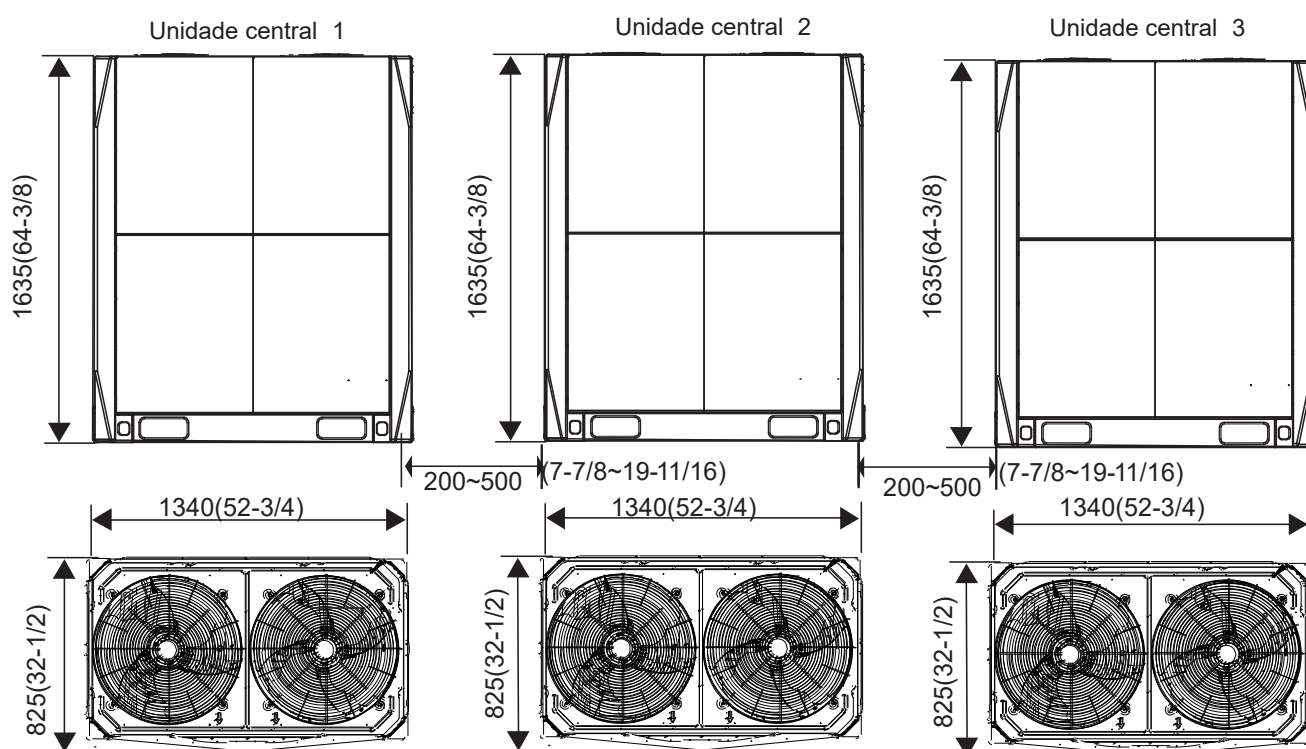
Figura 2-2.19: Dimensões da unidade 52/54/56/58HP (unidade: mm (polegada))
