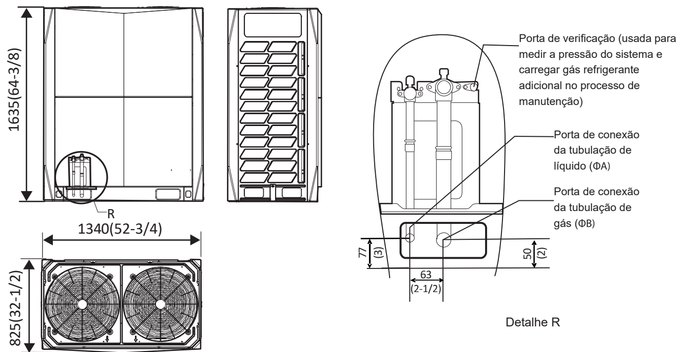
Figura 2-2.2: Dimensões 14/16/18/20/22HP (unidade: mm (polegada))
