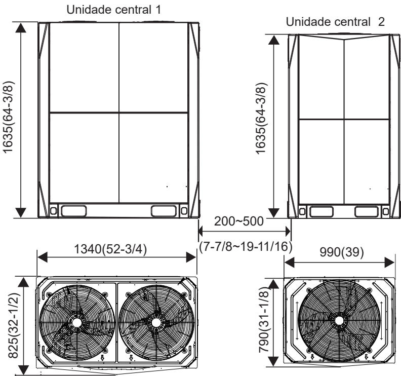
Figura 2-2.5: Dimensões da unidade 34HP (unidade: mm (polegada))
