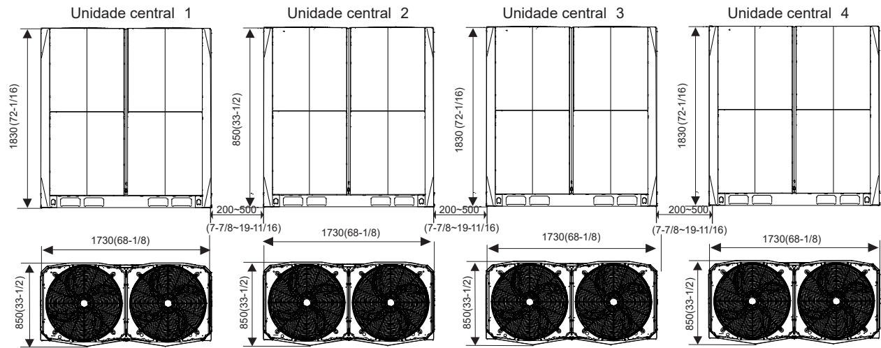
Figura 2-2.24: Dimensões da unidade 96*HP (unidade: mm (polegada))
