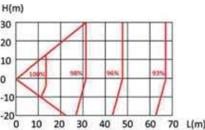
Figura 2-7.6: Taxa de alteração do modelo 38ATQA48 / 38ATQA56 na capacidade de aquecimento
