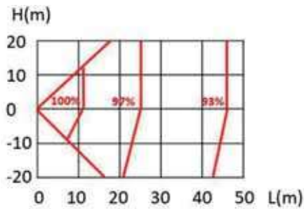
Figura 2-7.5: Taxa de alteração do modelo 38ATQA48 / 38ATQA56 na capacidade de refrigeração
