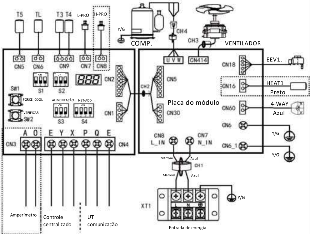
Figura 2-5.1: Modelo 38ATQA28
