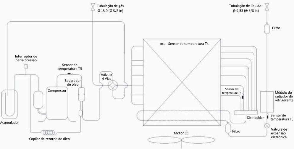
Figura 2-4.1: Modelo 38ATQA28
