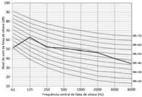
Figura 2-9.6: nível da faixa de oitava - 38ATQA56
