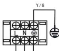
Figura 3-8.2: Terminais da fonte de alimentação monofásica da unidade central
